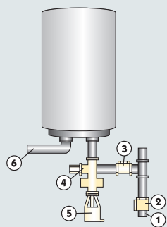
vertikaal wandmodel
