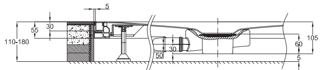
Afbeelding met afvoergarnituur BETTEFLOOR - 0,85 l/s, horizontale ontwatering normbepaalde waterstand 50 mm
