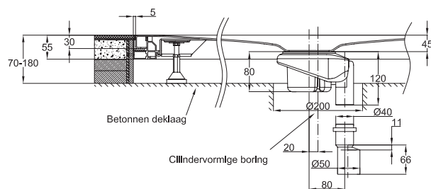
Afbeelding met afvoergarnituur - 0,6 l/s, verticale ontwatering normbepaalde waterstand 50 mm
