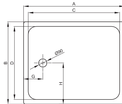
Douchebak met een muurlengte \geq 100 cm
