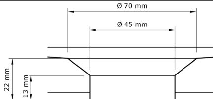
DETALLE ZONA DESAGÜE/DÉTAIL ZONE EVACUATION
