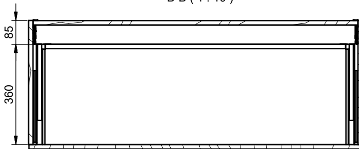
B-B (1 : 10)
